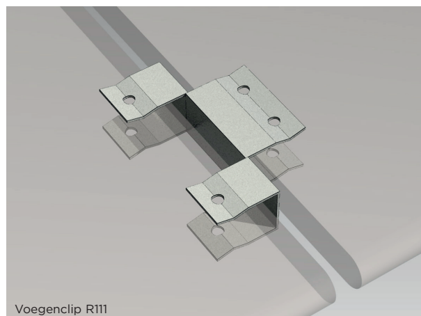
Voegenclip R111
