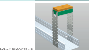
PlaGyp® PU60/125 dB
