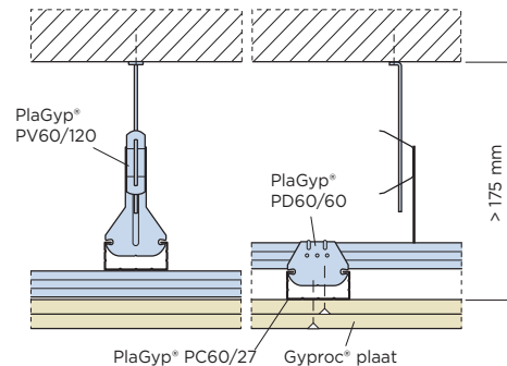
Bevestigen met Nonius
