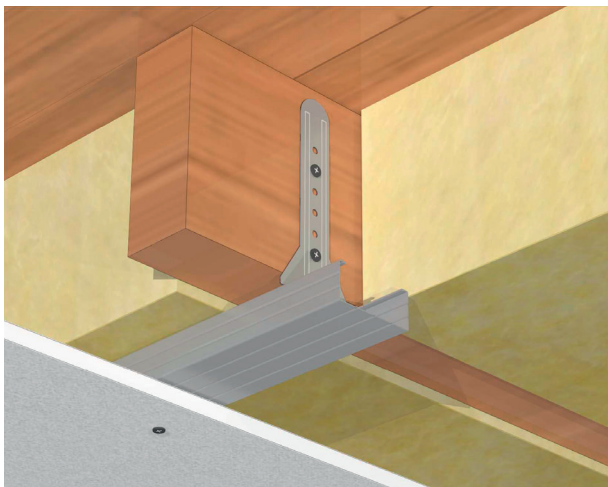
PlaGyp® plafond
