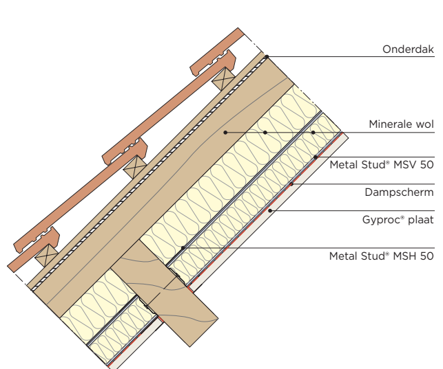
Snede Metal Stud® tussen gordingendak
