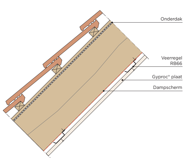
Snede veerregel onder spantendak
