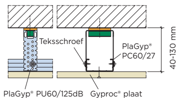
Bevestigen met PlaGyp® PU60/125dB
