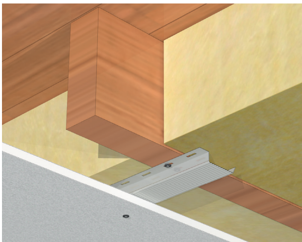
Veerregelplafond
