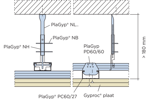
Dilatatievoeg
