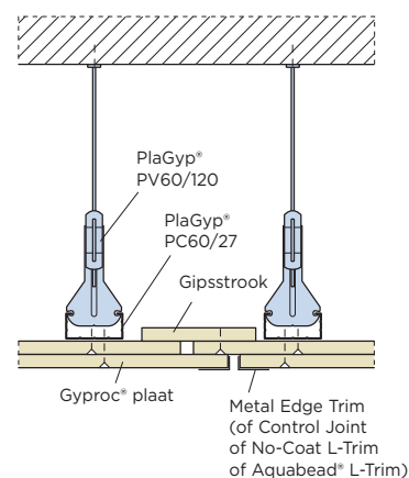
Dilatatievoeg
